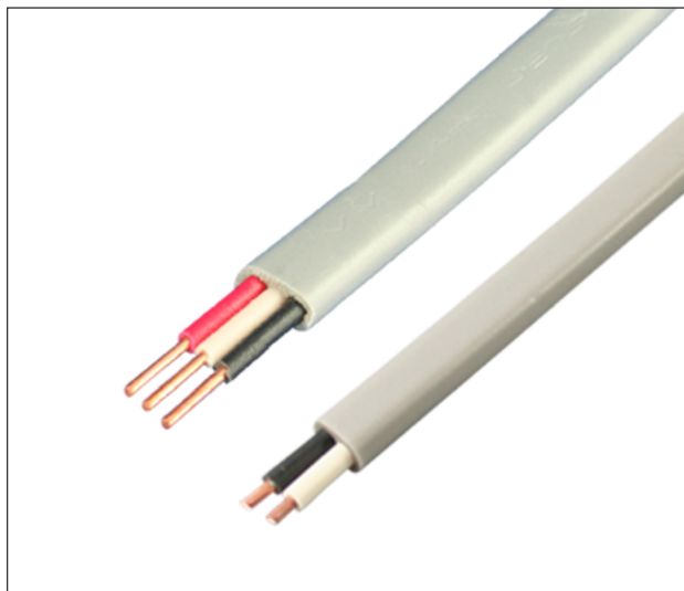
画像例：VVF 2.0mm × 2C 灰 ：VVF 1.6mm × 3C 灰
